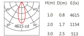
5050 45° RGBW(4000K)
