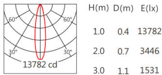
5050 20° RGBW(4000K)
